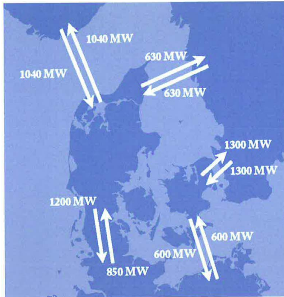
De danske kabelforbindelser
