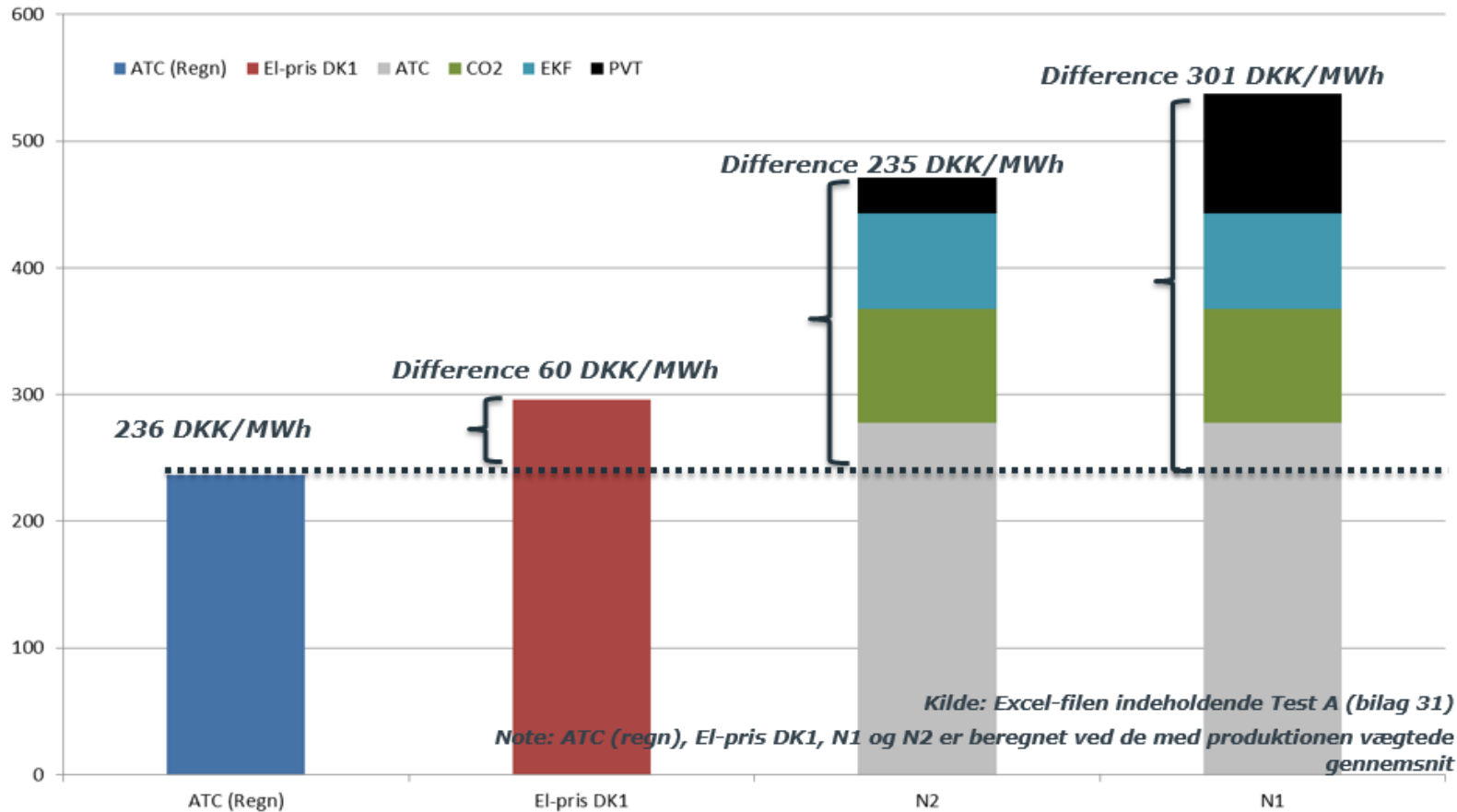
Sammenligning af ELSAM Kraft A/S' ATC(regnskab), el-prisen i DK1, 3-timers teststørrelsen (N1) og 10-timers teststørrelsen (N2) kun for 2005
